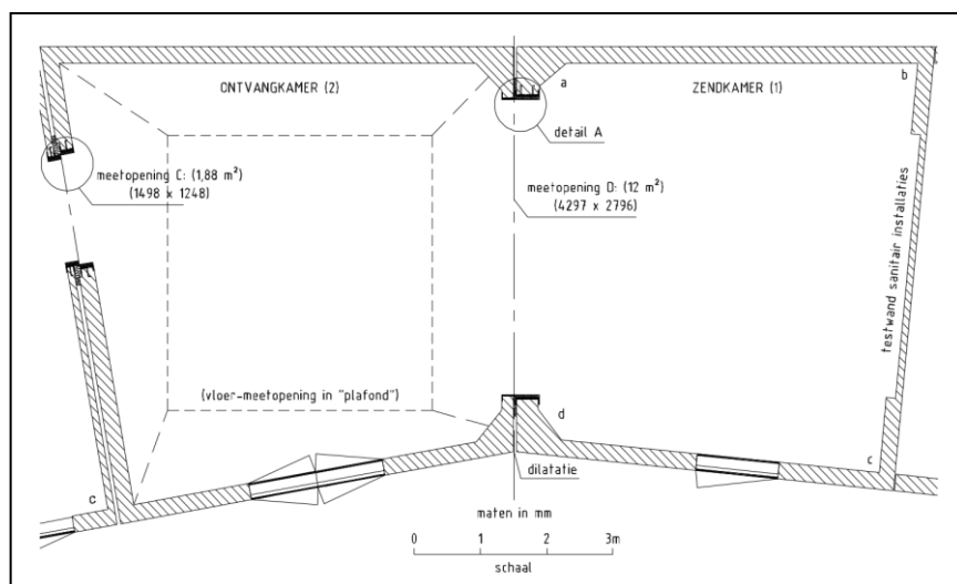
Figure 1 : Schéma des pièces de mesure du laboratoire PEUTZ nl
