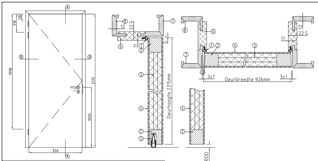
Figure 2 : Schéma test du détalonnage sur un bloc-porte
